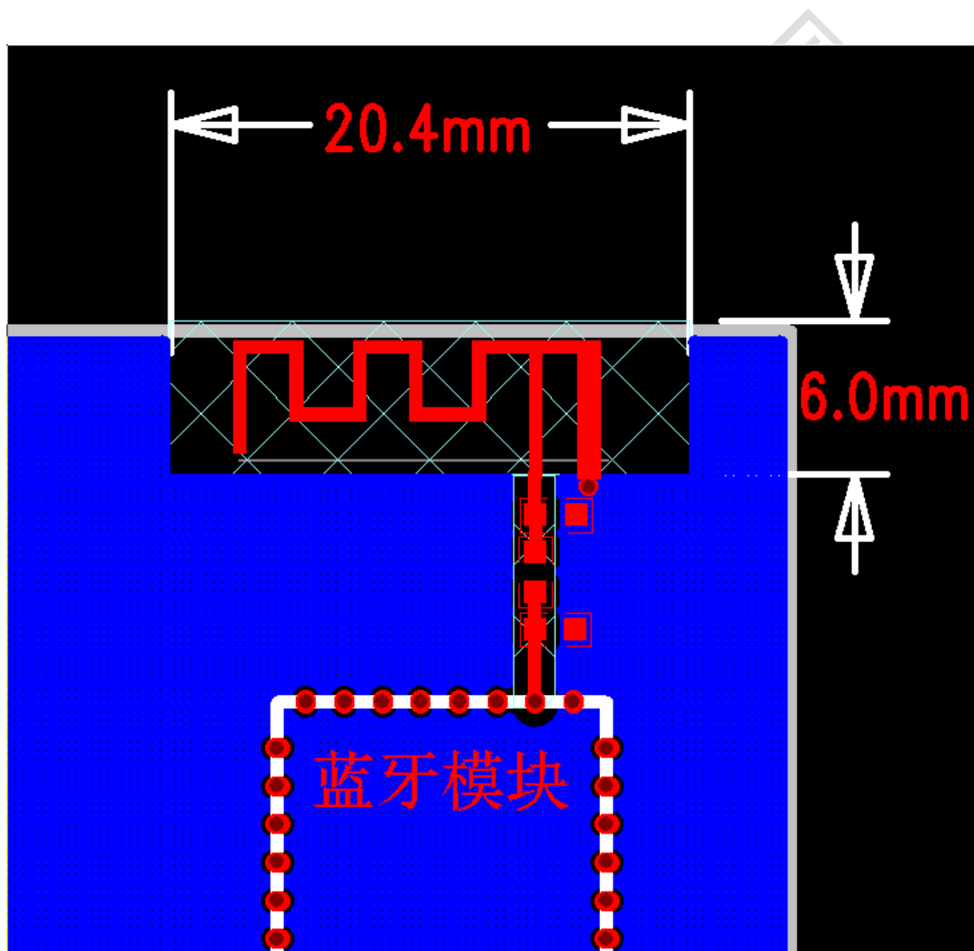
外置天线
