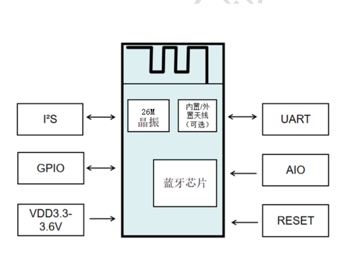
MY-BT201 框图(顶视图)
