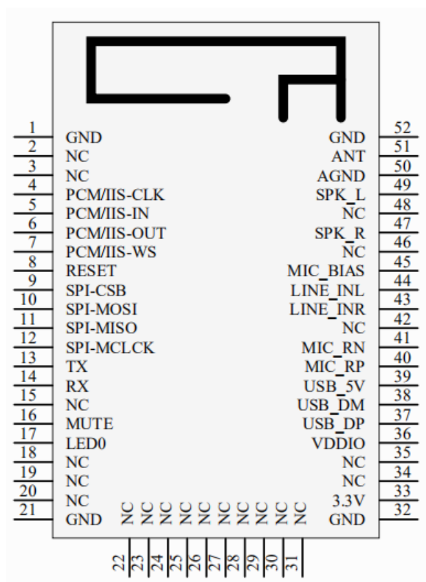
MY-BT201 引脚定义图(顶视图)
